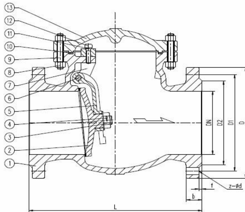
Рис.1 Клапан обратный подъемный фланцевый.
